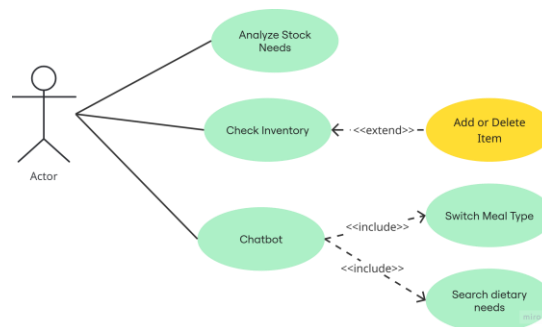
Gambar 3.4 Use Case Keseluruhan Aplikasi
