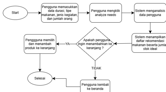
Gambar 3.2 Flowchart fitur analisis kebutuhan stok
